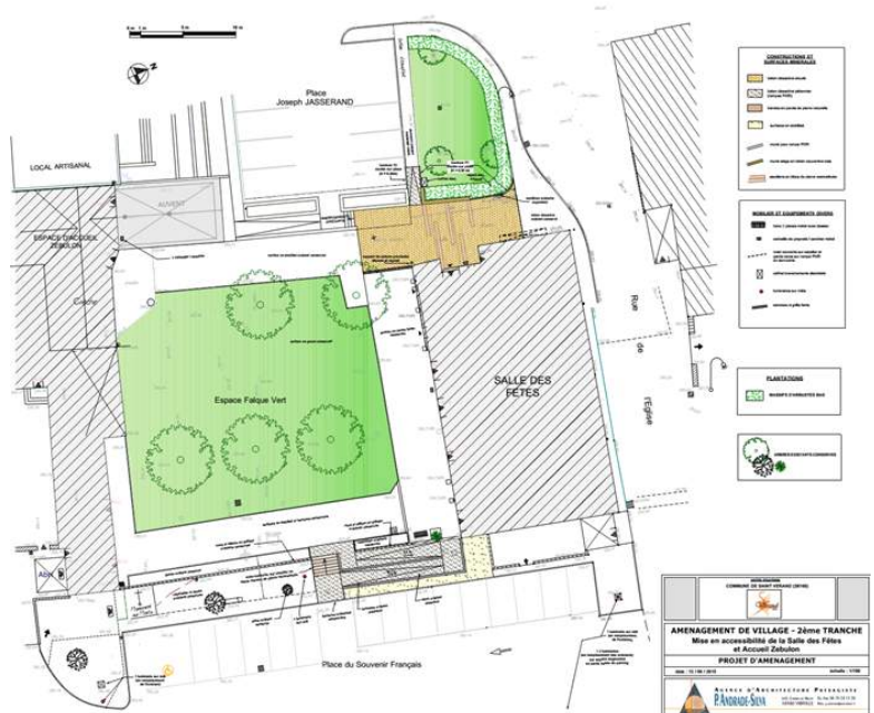
Plan de composition de l'aménagement avec reprise du parvis de l'entrée principale de la salle des fêtes et emplacement de la rampe d'accès coté parking de l'école.
